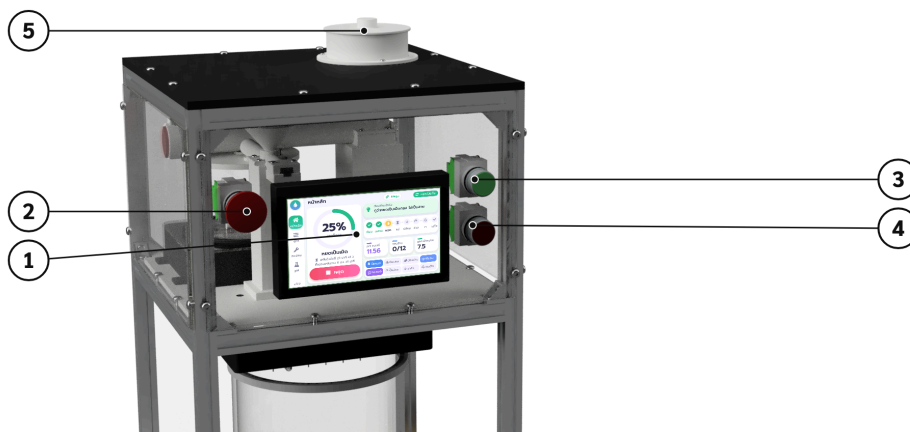
รูปที่ 1 แผงควบคุม: 1 จอ · 2 E-stop · 3 START · 4 STOP · 5 ฝาถังผง
